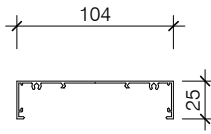
HAS010-A AS104 CAPPING HEAD/FRAME
