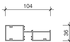
HAS021-A AS104 GLAZING SILL/TRANSOM
