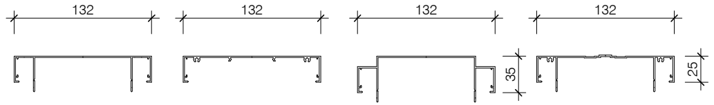
HAS310 AS132 HEAD/SILL TRACK
